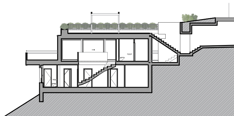
COUPE LONGITUDINALE VILLAS B
