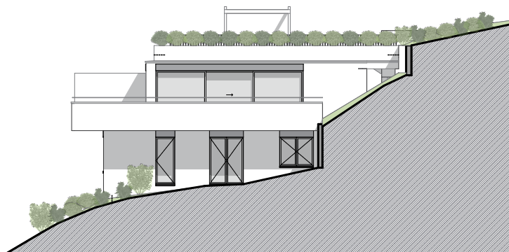
FACADE EST VILLAS B
