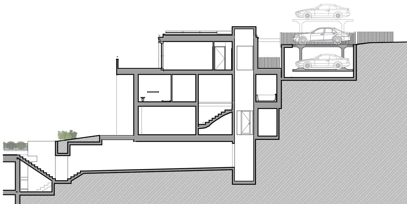
COUPE LONGITUDINALE BATIMENT A
